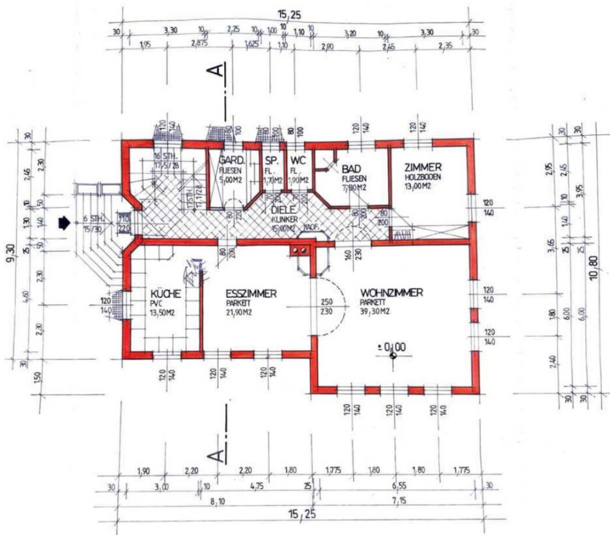
ERDGESCHOSS WNFL. 118,60 M 2
